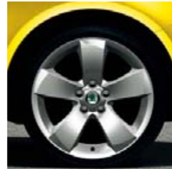
Kolo z lehké slitiny Kentaur 7,0J x 17" pro pneumatiky 205/40 R17 (5J0 071 496)
